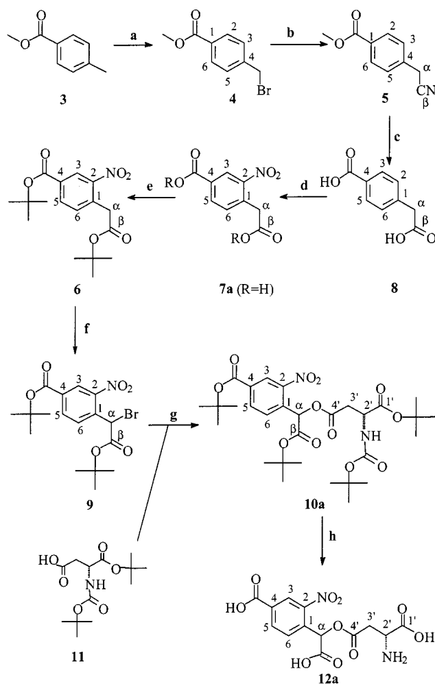
Scheme 2. Synthesis of \beta -( \alpha,4 -DCNB)-D-aspartate 12a . a: \text{Br}_2 , benzene, h\nu , 86 %, b: KCN, EtOH, \text{H}_2\text{O} , 74 %, c: \text{H}_2\text{SO}_4 , \text{H}_2\text{O} , 87 %, d: \text{HNO}_3 , \text{H}_2\text{SO}_4 , 70 %, e: isobutene, \text{H}_2\text{SO}_4 , 20 °C, \text{CHCl}_3 , 57 %, f: NBS, \text{CCl}_4 , 34 %, g: DBU, benzene 58 %, h: TFA, toluene, 88 %
